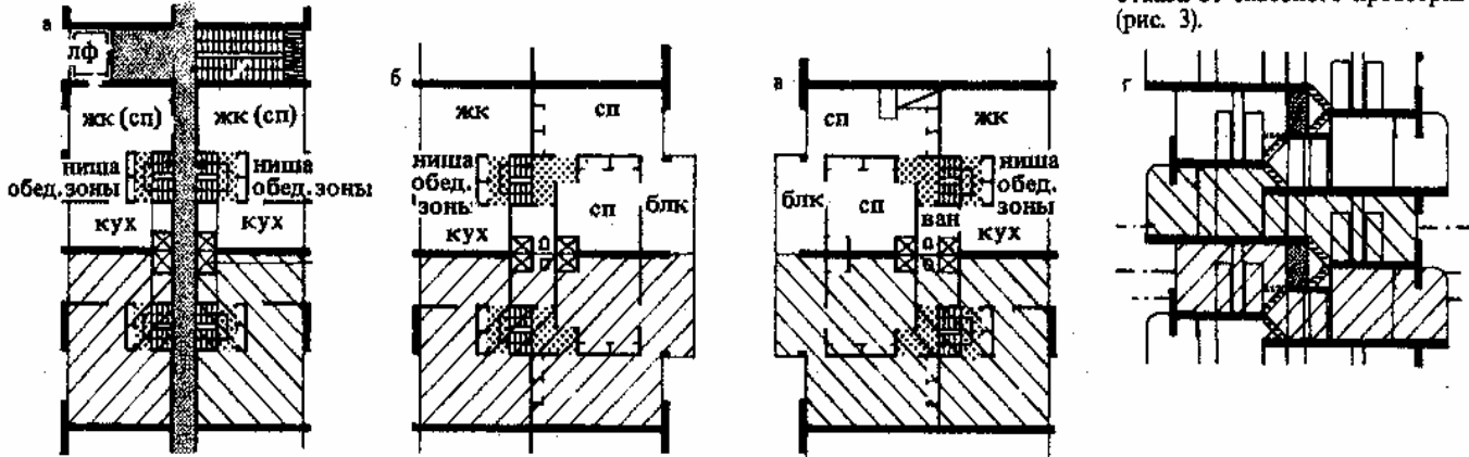
2. Многоэтажный жилой дом коридорного типа со смещенными уровнями полов. Окна каждой квартиры выходят на обе стороны дома (сквозное проветривание). Архит. Э. Нейферт
