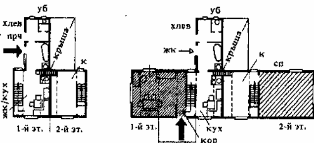
4. Двухквартирный дом, расширенный путем пристройки на уровне земли и надстройки (мансарды) над жилой комнатой. Архит. Таут
