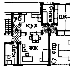
6. Трехкомнатная квартира с отдельной уборной для гостей и домашней работницы рядом с передней. Оптимальное расположение внутреннего коридора, точно соответствующее приведенной выше схеме (рис. 3). Архит. Э. Нойферт
