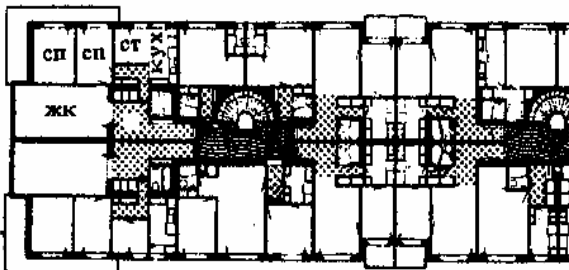
9. Типичный план секции жилого многоквартирного дома в Стокгольме с семью квартирами на одной лестничной площадке; квартиры одно-, двух-, трех и четырехкомнатные. Темные лестничные клетки, кухни и санитарные узлы расположены во внутренней зоне дома. Вентиляция — через воздушные продухи под окнами, количество пропускаемого воздуха регулируется. Вытяжка — через вентиляционные шахты. М 1:500.
