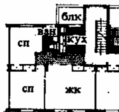
12. Трехкомнатная квартира с ванной комнатой и кухней, расположенными рядом с лестничной клеткой; по средней продольной оси дома размещены колонны, по которым уложены прогоны со шкафными стенками между ними. Архит. В. Р. Мак-Корнак
