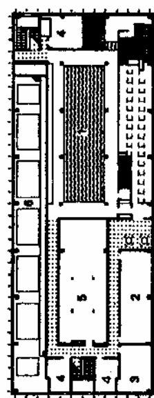
11. План на уровне 19-го этажа, Архит. Х. Штоль 1-плавательный бассейн; 2-гимнастический зал; 3-комната отдыха; 4-вентиляционная камера; 5-искусственный охладитель
