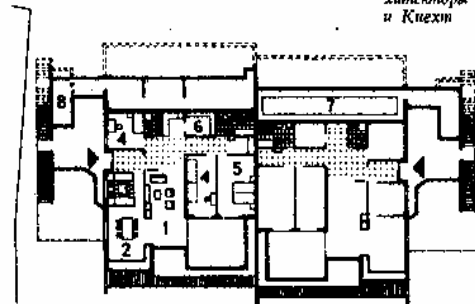
8. План террасного жилого дома. Архитекторы Штуки и Мекен
