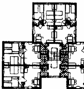
7. Шестиквартирная секция. М 1:500. Архит. Р. Ладеви
