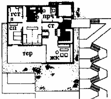
2. Частичное включение свободного пространства (части открытой террасы) в основной объем дома
