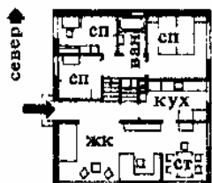
3. План дома со смещенными этажами (Дания). В проекте предусмотрены хорошие взаимосвязи между спальнями и общей комнатой. Архит. С. Мортенсен
