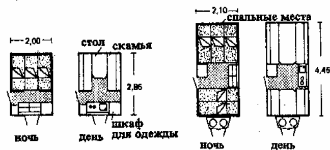
8. Вагон-домик с тремя кроватями и встроенным кухонным оборудованием
