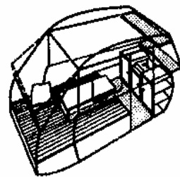
13. Перспектива автоприцепа, изображенного на рис. 12, с показом деталей интерьера. Ночью — на месте, занимаемом столом, раскладываются три спальных места
