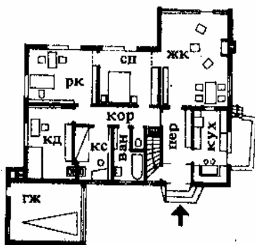
3. Квартира для семьи из 4 чел.; в подвале размещаются кладовая, котельная, прачечная и кладовая. Архит. Нойферт
