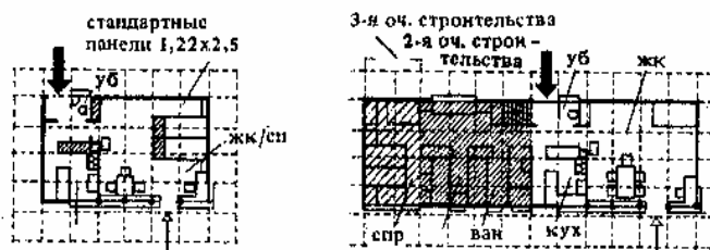
1. Одностороннее расширение дома, простейшее увеличение посредством удлинения. Торговая стена при расширении разбирается и панели используются вторично. Конструкции стен, выполняемые из одинаковых панелей обуславливают применение унифицированных размеров и кратность размеров всех помещений одному модулю. Архитекторы Жаскар и Кантала
