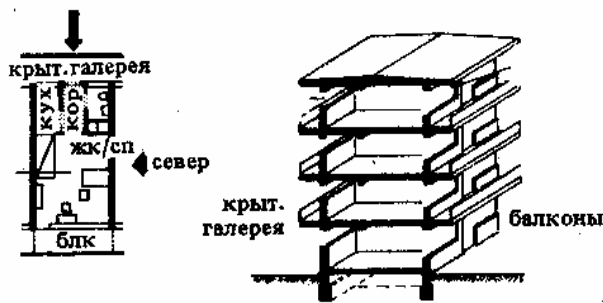
1. Франкфуртский тип квартиры в жилом доме с крытыми галереями, с непрерывным балконом, устроенным на солнечной стороне дома
