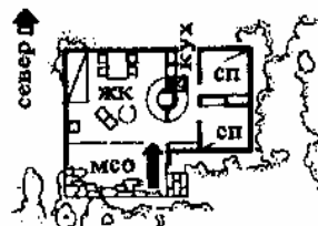
4. Дача с двумя спальными местами, местом для приготовления пищи, гардеробом для одежды, крыльцом и каминком в жилой комнате. Архитекторы Хитнен и Луукконен
