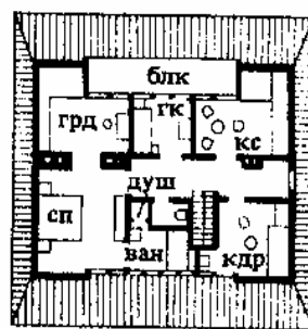
9. План 2-го этажа к рис. 8
