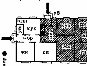
10. Разделение посредством закрытия одной из дверей, дом разделен на неравные части
