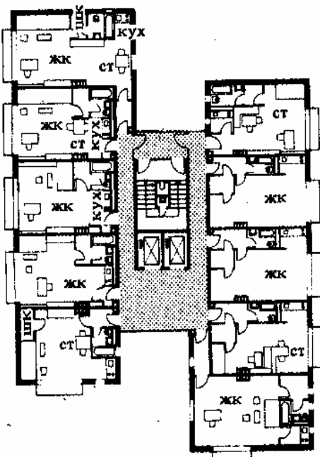
4. Односекционный жилой дом гостиничного типа, на каждом этаже по 10 квартир, причем планировка квартир варьируется. В западном блоке предусмотрены шкафы с кухонным оборудованием, в восточном блоке — кухонные ниши. Архитекторы Мюллер-Рем, Зигмани
