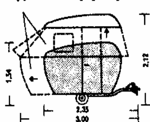
12. Небольшой жилой автоприцеп, во время движения компактно сложенный и закрытый, раскрываемый на стоянке. Включает в себя спальный отсек, отсеки для отдыха и приготовления пищи, а также багажные
