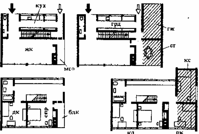
5. Отдельно стоящий одноквартирный дом, расширенный путем пристройки в связи с достижением детьми совершеннолетия, предусмотрено крыльцо с местом для отдыха, а над ним балконная плита, служащая консольной опорой для навешиваемого позже перекрытия
