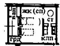
14. Американская планировка квартиры в доме коридорного типа с вытяжной вентиляционной шахтой в небольшой кухне. Кухня освещена вторым светом через столовую
