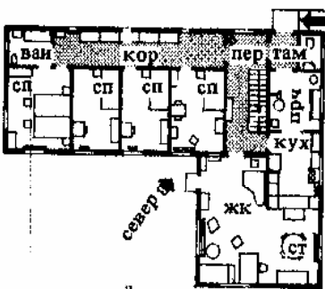
5. Жилой дом углового очертания в плане, разделенный на два крыла для дневного и ночного пребывания. Крыло для дневного пребывания решено аналогично (рис. 2). Архитекторы Кесслер и Петер, г. Юрих
