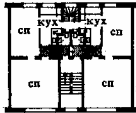
4. Типичный план датского секционного многоквартирного жилого дома со специальной холостой лестницей, предусматриваемой даже в самых малогабаритных квартирах. Уборная освещена вторым светом. Вытяжные устройства см. с. 224
