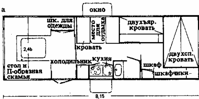
7. Большой жилой вагон-домик на 8-9 спальных мест (а), на 6-7 спальных мест (б и в)
