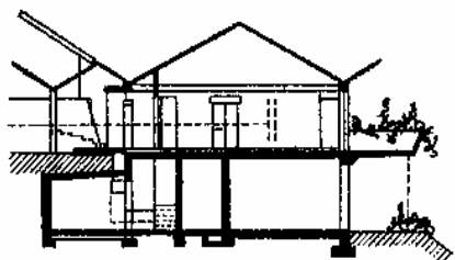
7. Нижний этаж
