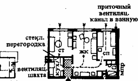
13. Обычная трехкомнатная квартира с направлением потока свежего воздуха от окон к вытяжной вентиляционной шахте. М 1:400
