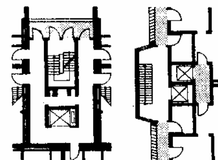
6. Две лестничные клетки с лифтами и мусоропроводами. В хозяйственные зоны квартир предусмотрен проход по вспомогательным лестницам с промежуточной площадки. Зап. Берлин. Архит. Палец-Бодуэн. М 1:300
