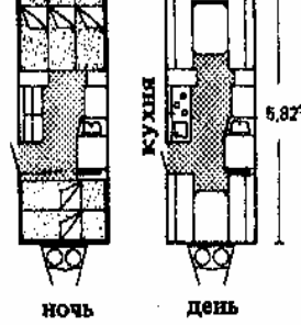
11. Вагон-домик с пятью кроватями, туалетом и раздвижной перегородкой
