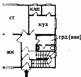
15. Чем лучше пространственная связь передней и лестницы, тем лучше пространственная связь между первым и вторым этажами
