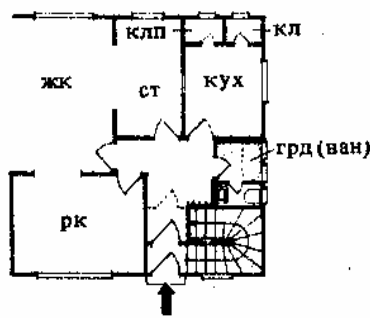
13. Неправильно такое расположение угловой лестницы, когда ее фризовая ступень находится в тамбуре и лестница пространственно чрезмерно отделена от передней
