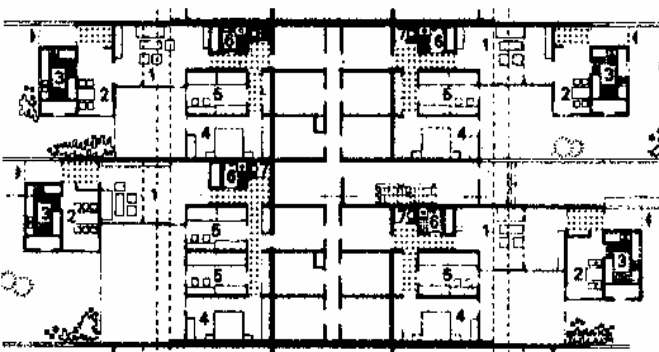
10. План 1-го этажа террасного жилого дома — «холма». Архитекторы Фрей, Шредер, Шмидт
