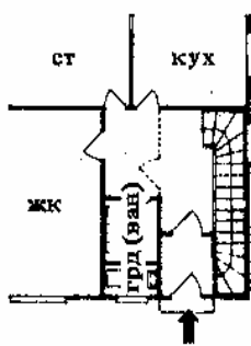
18. Предпочтительна планировка с устройством просторной гардеробной, которая после разделения дома на две квартиры переоборудуется в ванную
