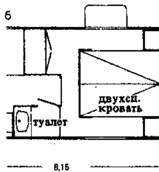
6. Лодка-домик для отдыха в выходные дни. Софа может откидываться вверх, как вторая вагонная полка (см. с. 214, рис. 12), в результате чего в домике получается 6 спальных мест. План и разрез. Архит. Ф. Форбс
