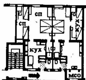
15. Жилой дом с короткими галереями, на две квартиры (всего на лестницу четыре квартиры). Душевая освещается вторым светом и проветривается через светлое помещение уборной. Встроенные шкафы в кухне и передней. М 1:400. Архит. Р. Фридман
