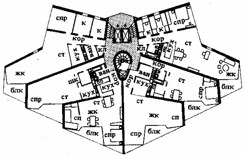
3. Односекционный дом южной ориентации с шестью квартирами на каждом этаже. Кухни, санитарные узлы расположены в средней зоне дома, оснащены искусственной вентиляцией и проветриваются при сквозном проветривании квартиры. Кабины лифта останавливаются на промежуточных лестничных площадках. Вторая лестница — темная, винтовая. М 1:400. Архит. Лембрах
