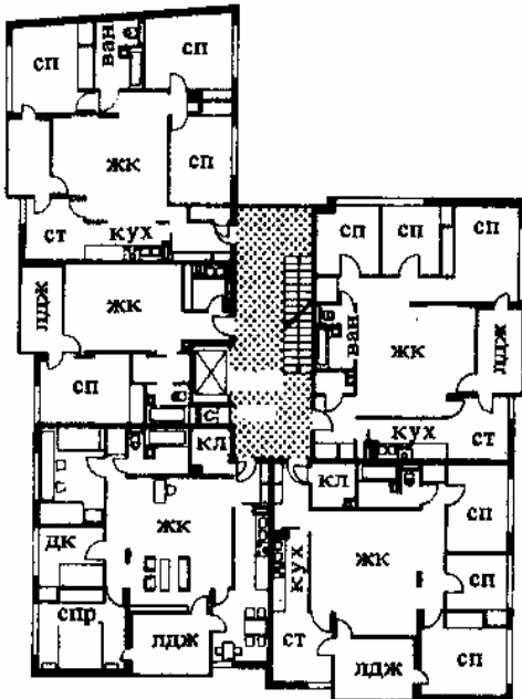
8. Односекционный дом с пятью квартирами на этаже. Лестница размещена в глубокой лоджии. Общая комната-проходная. Зап. Берлин. М 1:400. Архит. Аалто
