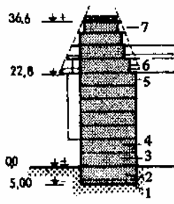
3. Поперечный разрез здания «Чилихаус» в г. Гамбург. Архит. Ф. Хегер
