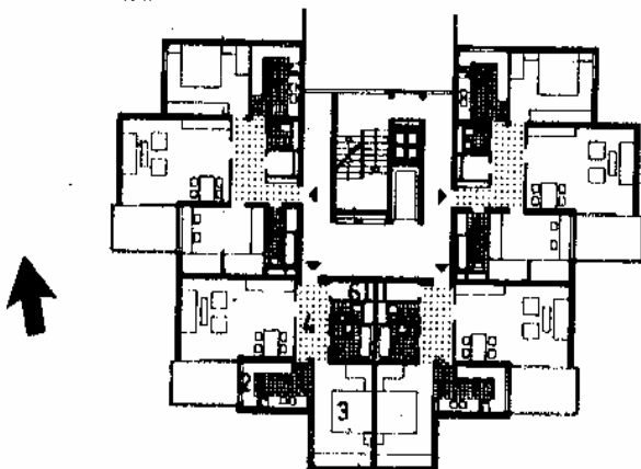
1-жилая комната; 2-кухня; 3-спальня; 4-коридор; 5-ванная; 6-кладовая
