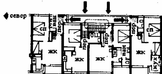
4. Эта планировка предусматривает зрительную изоляцию квартиры путем понижения отметки пола крытой галереи на две ступени по отношению к отметке пола квартиры. План и разрез. Архит. Ф. Лебеллер
