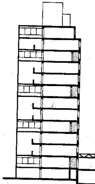
14. Галерейный дом системы «Триплекс». Крытая галерея располагается на каждом третьем этаже. В большие квартиры ведут отдельные входы с внутриквартирными лестницами. Все квартиры имеют сквозное проветривание. М 1:200. Кембридж, США. Архит. Кох-Кеннеди
