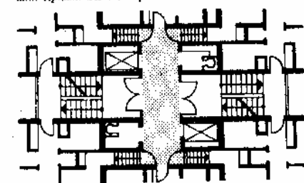
6. Две лестничные клетки с лифтами и мусоропроводами. В хозяйственные зоны квартир предусмотрен проход по вспомогательным лестницам с промежуточной площадки. Зап. Берлин. Архит. Палец-Бодуэн. М 1:300
