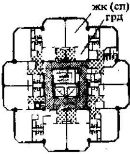
1. Небольшие квартиры (в доме гостиничного типа), расположенные вокруг коммуникационно-транспортной шахты в односекционном 16-этажном доме. М 1:1000, Архит. Ример, Вашингтон
