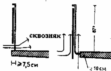
10. Ограждение балкона опущено ниже и вынесено за пределы балконной плиты в плане
