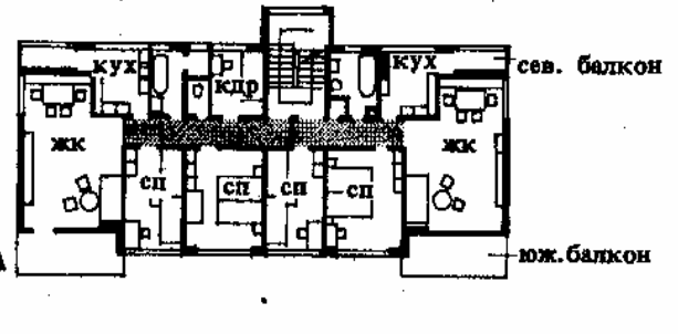
9. Двухкомнатная квартира со смежной межквартирной перегородкой, позволяющей расширить однокомнатную квартиру и превратить ее в двухкомнатную, со смежными комнатами. Такому решению присущи только недостатки. Архит. Н. Г. Фриберг
