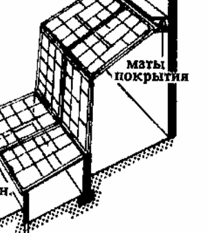
16. Теплица из парниковых рам, пристроенная к стене дома
