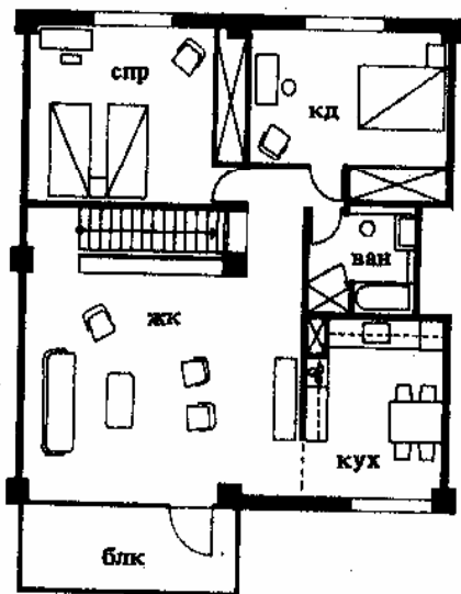
14. Галерейный дом системы «Триплекс». Крытая галерея располагается на каждом третьем этаже. В большие квартиры ведут отдельные входы с внутриквартирными лестницами. Все квартиры имеют сквозное проветривание. М 1:200. Кембридж, США. Архит. Кох-Кеннеди
