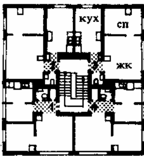
6. Датская планировка односекционного дома с четырьмя двухкомнатными квартирами с входами с основной и промежуточной площадок лестницы
