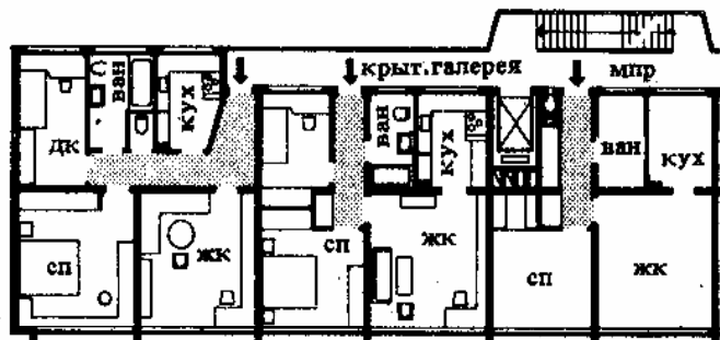
5. Проход в кухню — через жилую комнату; исключения представляют лишь квартиры, расположенные в торца дома. Ванная, кухня, уборная объединены в общий санитарно-технический блок
