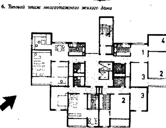
1-столовая; 2-жилая комната; 3-спальня; 4-детская
