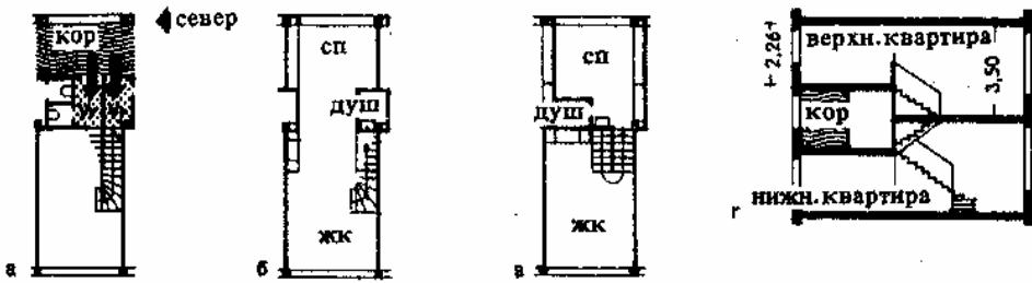
1. Русский тип квартиры. Малометражные квартиры со спальнями пониженной высоты и высокими общими комнатами. Наружный коридор обслуживает два этажа. Уборная без естественного освещения примыкает к передней. Архит. М. Я. Гинзбург, Москва
