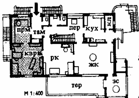
5. Большой многоквартирный жилой дом близ Хельсинки. М 1:400. Архит. Аарне Эрви
