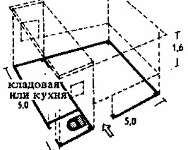
7. Помещение овощной отделено палаточным брезентом. Нижняя часть помещения - из массивных конструктивных элементов
