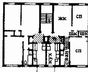
5. Типичный план американской квартиры с неудачным расположением внутреннего коридора. Архит. Слейн
