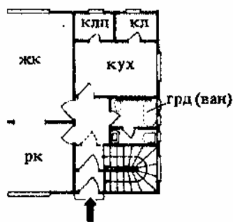
14. Планировка помещений одноквартирного дома требует хорошей пространственной связи между передней и лестницей; фризовая ступень лестницы должна находиться в передней
