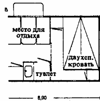
6. Лодка-домик для отдыха в выходные дни. Софа может откидываться вверх, как вторая вагонная полка (см. с. 214, рис. 12), в результате чего в домике получается 6 спальных мест. План и разрез. Архит. Ф. Форбс
