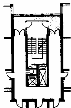
4. Лестничная клетка, лифты и мусоропровод объединены в компактное ядро. Площадки лестничной клетки отделены от коридора двойными дверями (дымопроницаемые отсеки). Зап. Берлин. Архит. Хассенфлуз. М 1:300
