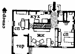
1. Жилой дом для бездетной супружеской четы; расположенная в центре лестница ведет на чердак и в подвал. Удачное взаиморасположение столовой и кухни, жилой комнаты и террасы. Архитекторы Эрмандорфер и Киндлер
