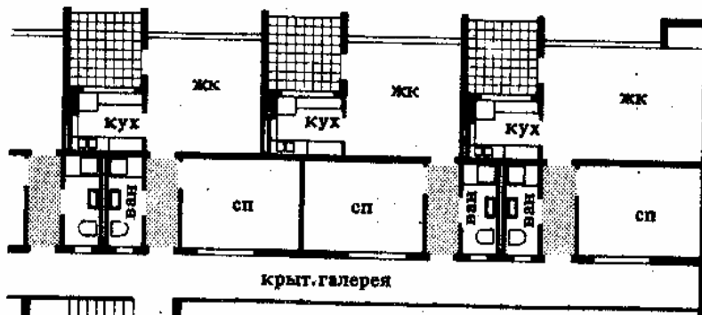
16. Лестничная клетка пристроена к галерее. Кухни освещаются через лоджии. Совмещенные санузлы оборудованы сидячими ваннами М 1:250. Архит. Зейтц
