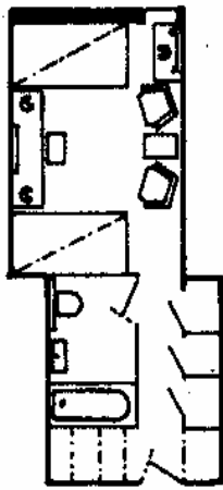
2. Двухместная каюта с двумя нижними койками, уборной и ванной
