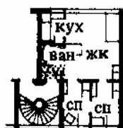
8. Шведская трехкомнатная квартира; кухни и ванные двух смежных квартир облокированы в зоне лестничной клетки. Архитекторы Н. Арбом и Х. Цимдал
