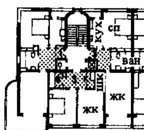
12. Трехквартирная секция с двухкомнатными квартирами, и помещения для счетчика на лестничной площадке. Архит. М. Бройлард
