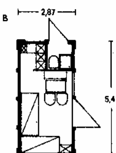
11. Дача из сборных конструктивных элементов с шагом планировочной сетки 1,25 м. Жилая площадь 36,4 м². Архит. Х. Дамм
