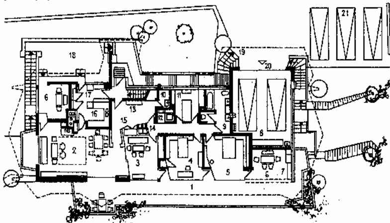
6. Жилой дом в Бумбурге, 1963 г. Верхний этаж. Архит. Нойферт
