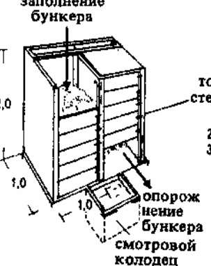
12. Бункер для удобрений
