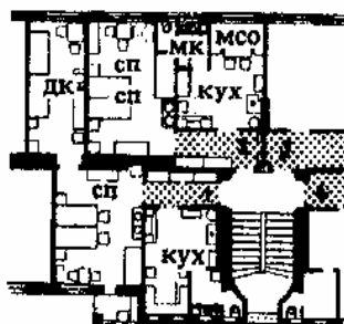
16. Венский тип секций: двухкомнатные и однокомнатные квартиры с кухней-столовой
