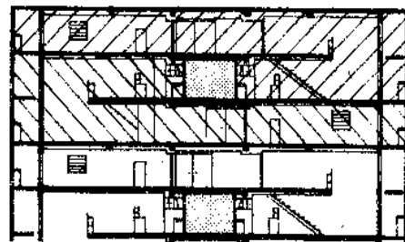
3. Малометражные квартиры в доме с одноканальными лестницами по центральной проходной оси здания (с верхним светом). С площадок лестницы входы в две квартиры со сквозным проветриванием. Архит. Э. Нейферт, 1934 г.
