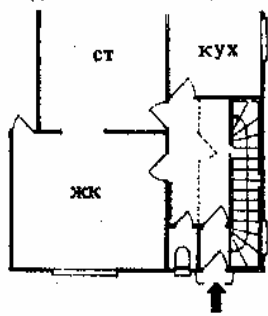
17. Неправильным является устройство одномаршевых угловых лестниц в тех случаях, когда при разделении дома на две квартиры, передняя разделяется длинной стеной на два узких длинных помещения
