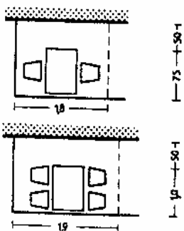
12. Необходимые размеры при размещении стола и стульев
