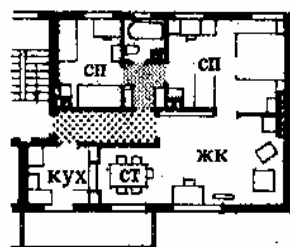
2. Трехкомнатная квартира с отдельным коридором между спальнями и ванной комнатой. Архит. А. Клейн
