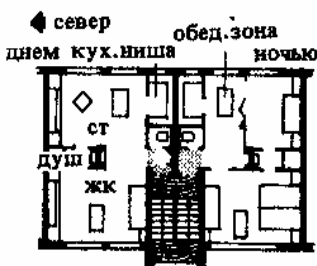
11. Трансформируемая квартира с постоянно используемыми помещениями (днем и ночью) благодаря наличию убиралочных или поворотных кроватей, складывающихся перегородок и т. п. (общая площадь — 40 м 2 ). Архит. К. Фигер, Зап. Берлин
