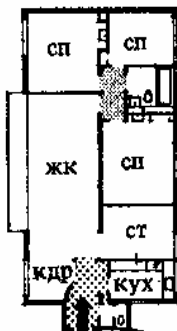
4. Современная английская пятикомнатная квартира с удачной компоновкой помещений и внутреннего коридора. Архит. Либеткин
