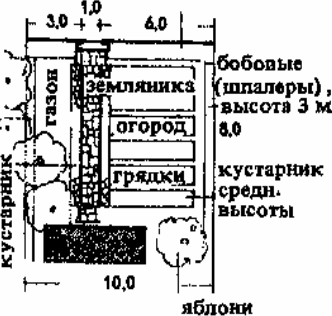
2. Земельный участок площадью 120 м² в районе Вестфридгоф в г. Мюнхен. Архит. Харберс
