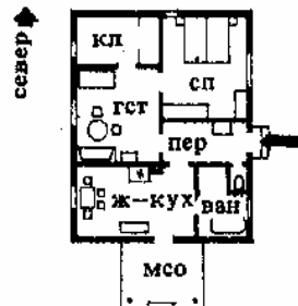
2. Жилой дом садовника с кухней-столовой. Архит. Вернер
