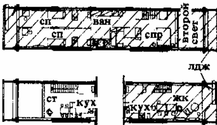
3. Малометражные квартиры в доме с одноканальными лестницами по центральной проходной оси здания (с верхним светом). С площадок лестницы входы в две квартиры со сквозным проветриванием. Архит. Э. Нейферт, 1934 г.
