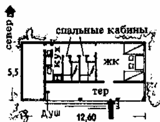
7. Дача и база отдыха на оз. Цугер Зее, рассчитанная на пребывание 6 чел. В спальнях кабинках-двухъярусные кровати. Через уборную-проход в помещение гаража. Душевая расположена на террасе, обращенной к озеру. Архитектор Х.Р. Бек и К. Моссдорф
