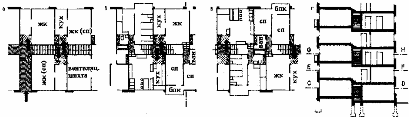
3. Малометражные квартиры в доме с одноканальными лестницами по центральной проходной оси здания (с верхним светом). С площадок лестницы входы в две квартиры со сквозным проветриванием. Архит. Э. Нейферт, 1934 г.
