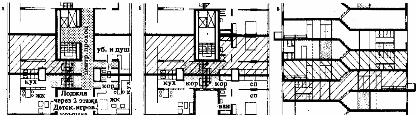
5. Положение центрального коридора в плане переменное. Коридор короткий, хорошо освещенный; одноканальные лестницы размещены на уровне коридора, в трехкомнатных квартирах нужно подниматься (или спускаться) по коротким внутриквартирным лестницам. М. 1:400. Архит. Ван де Брёк
