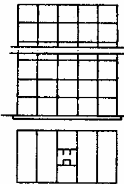
2. Конструктивный тип здания с поперечными стенами и ядром (конструктивное решение с использованием диафрагм)
