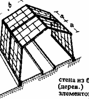
15. Теплица голландского типа со стенами из парниковых рам
