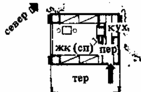
5. Однокомнатная дача с встроенными двухъярусными кроватями для четырех или восьми человек, с передней и изолированной кухней. Архит. В. Лейстен
