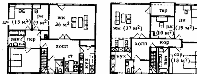
6. Дом из сборных конструктивных элементов с гибкой планировкой на основе планировочной сетки с ячейками 1,25 x 1,25 м
