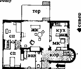
1-й этаж
