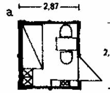
13. Садовый домик из сборных железобетонных элементов. Шаг планировочной сетки 1,23 м. Возможно строительство домиков шириной 3,9 м и длиной до 15,25 м. Жилая площадь: а-7,34 м²; б-10,57 м²; в-13,81 м²; г-17,04 м²
