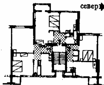
13. Трехквартирная секция с двухкомнатными квартирами, с развитым периметром наружных стен (улучшение изоляции и освещения квартир). Архит. Х. Мертенс
