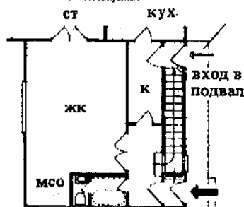
21. Благодаря смещению части стены и самой нижней ступени появляется возможность полного отделения перегородкой марша, ведущего в верхнюю квартиру. Вход в подвал для жилищной верхней квартиры совмещается с вспомогательным входом в нижнюю квартиру
