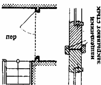
29. Перегородка, отделяющая коридор, устраивается из двух слоев с петлей и состыкованных дверей; шлик закрывается двумя нащельниками, закрепленными винтами
