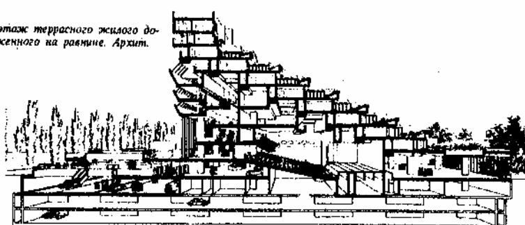
13. Поперечный разрез по зданию Центра конгрессов. Проект Е. Г. Зеля
