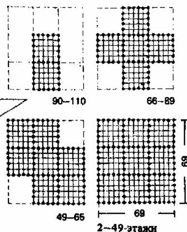
2-49-этажи
