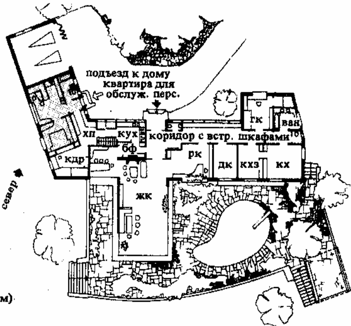
2. Одноэтажный жилой дом с квартирой шофера при нем. М 1:500. Архит. Нойферт (проект 1948 г.)
