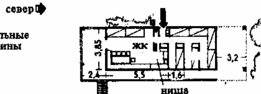
9. Дача на 8 или 16 чел. с открытой нишей для приготовления пищи. Жилая комната обращена окнами в сторону горного склона Базельской Юры. Архит. П. Артария
