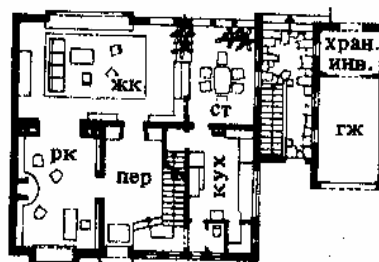
8. Хорошая взаимосвязь между передней и лестницей; кухня и столовая расположены на две ступени выше остальных помещений 1-го этажа. Архит. Финнер
