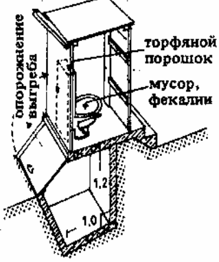
11. Выгребная уборная с засыпкой сухого торфа
