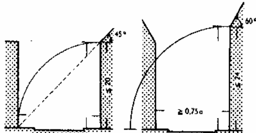
1. Зависимость между минимальной шириной улиц и высотой зданий в жилых кварталах (слева) и в промышленных и деловых кварталах (справа)
