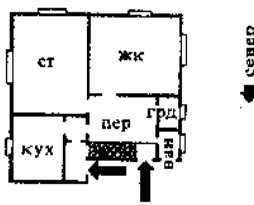
4. Типичное решение планировки дома с идущей вдоль стены лестницей. Для жильцов нижней квартиры нет лестницы, ведущей на чердак. Доступ в подвал для жильцов верхней квартиры — снаружи
