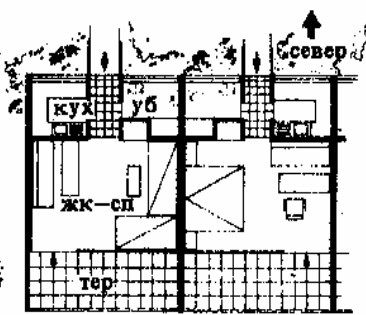
9. Дача на 8 или 16 чел. с открытой нишей для приготовления пищи. Жилая комната обращена окнами в сторону горного склона Базельской Юры. Архит. П. Артария
