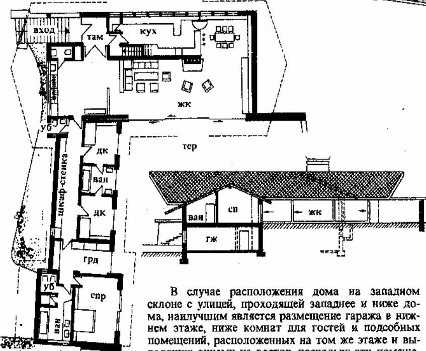
4. Жилой дом в г. Мильтенберг, 1963 г. План 1-го этажа и поперечный разрез
