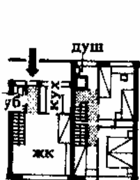
9. Франкфуртский тип жилого дома с крытыми галереями, с квартирами в двух уровнях. Второй этаж квартиры консольно выступает над находящейся под ним крытой галереей. План нижнего и верхнего этажей и разрез
