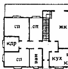
7. Дом с мансардой, занимающей половину чердака; вход в мансарду по лестнице из жилой комнаты
