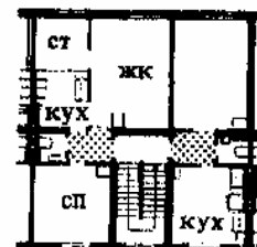
10. Современная планировка шведской двухквартирной секции: однокомнатная и двухкомнатная квартиры. Расположение кухни и ванной аналогично рис. 8. Архит. К. Мезин
