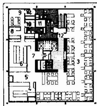
13. Типовой этаж. Здание Финн Ландхауз, г. Гамбург. Архитекторы Х. Хейнрих и Х. Печини 1-шахта коммуникаций инженерного оборудования; 2-конторское помещение; 3-ресторан; 4-буфет; 5-проход к шахте, соединенной с подвалом; 6-кухня; 7-гардероб; 8-кладовая для хранения древесного запаса продуктов; 9-холл; 10-помещение для персонала; 12-телефон
