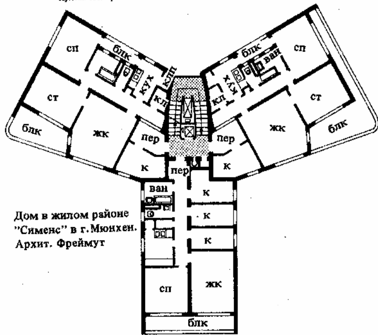
5. Высотный дом-трилистник с хорошей инсоляцией помещений при зрительной изоляции от других квартир, поскольку угол между блоками «трилистника» равен 120°. Возможно объединение нескольких таких жилых домов в дом рядовой застройки или же в казачий в плане дом (г. Кладно, ЧССР; Нью-Йорк, США). М 1:400, Архит. Фреймут
