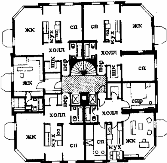
2. Шведский жилой дом башенного типа с темной лестницей. Исследовательская комиссия Строительного управления г. Стокгольма разработала по данной тематике 2000 чертежей планов М 1:400
