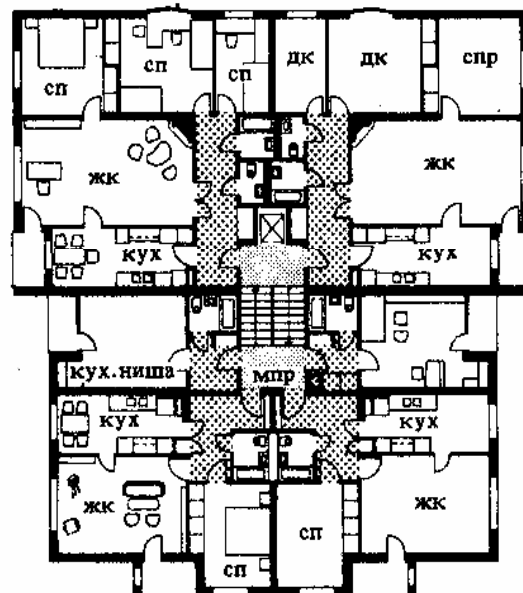
10. Односекционный жилой дом с шестью квартирами на разных уровнях. На каждой площадке темной лестницы, расположенной во внутренней зоне дома, находятся входы в квартиры. Мусоропровод с загрузкой с лестничной площадки, как и на рис. 4. М 1:400. Архит. Штреленорт, Стокгольм
