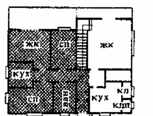
8. После разделения дома жилая комната с кухней, а также вспомогательное помещение отходят к квартире-мансарде
