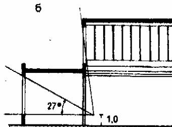
8. Шедовое или пилообразное покрытие создает более равномерную освещенность благодаря отражению света нижней поверхностью; при светлых крышах равномерность освещения повышается. Фонари не доводят до наружных стен здания
