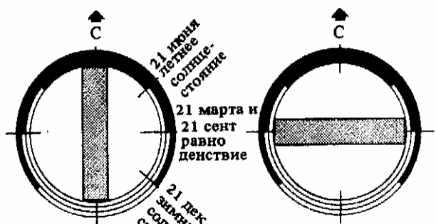
7. Широтная ориентация здания наиболее пригодна для квартир в 1-2 комнаты; на юг ориентируют общую комнату и спальню, на север - лестничную клетку, ванную, прихожую, кухню и т.д.
