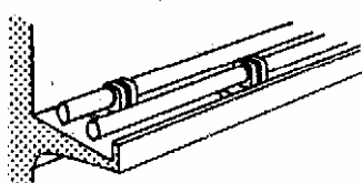
2. Размещение ламп вразбежку в двухламповом светильнике
