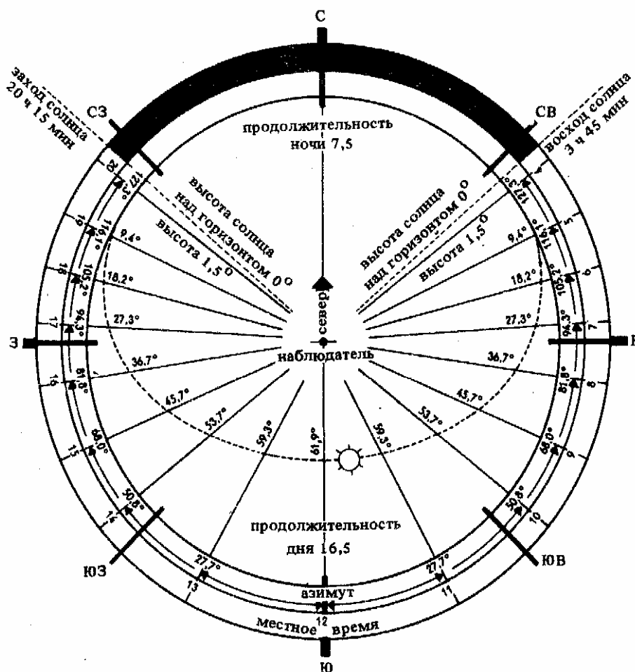
1. Траектория движения солнца в период солнцестояния (около 21 июня) для самой продолжительного дня в году ( 51,5^\circ северной широты, Дортмунд–Галле)
