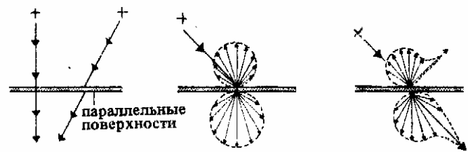
6. Направленное пропускание света прозрачными стеклами со смещением при кривых лучах
