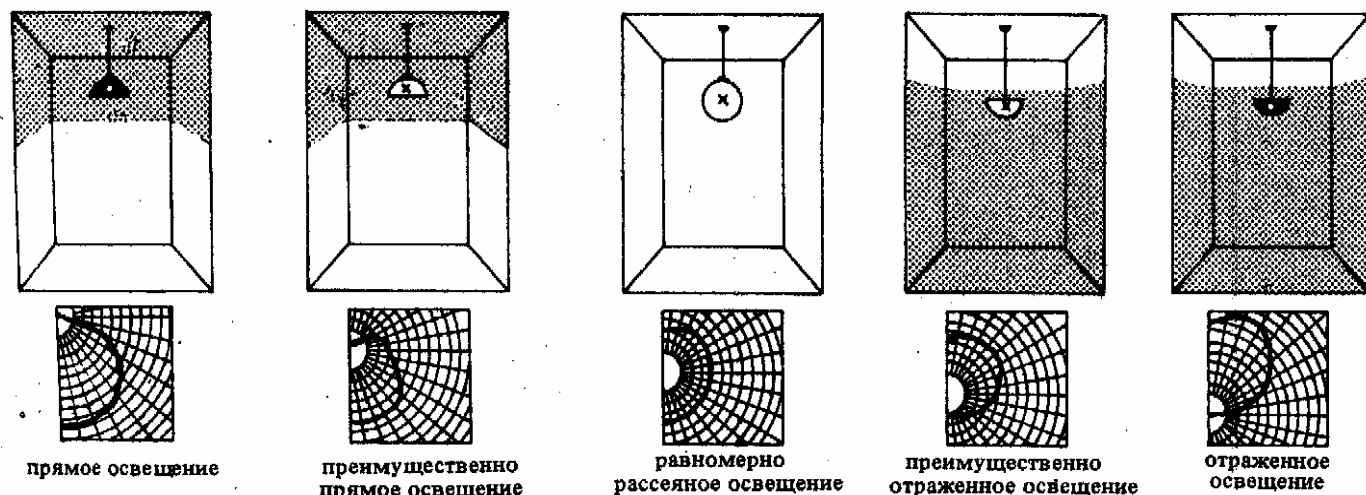
2. Стандартное распределение светового потока в зависимости от типа светильников
