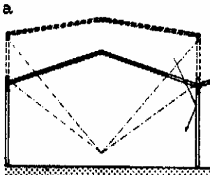
7. В одноэтажных зданиях наклонное остекление верхнего света экономнее вертикального. М-образные фонари (б) наиболее выгодны в связи с хорошим отражением света и обеспечением аэрации помещения
