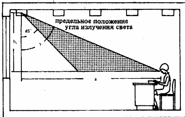
4. Диапазон излучений светильника, в котором должна выдерживаться предельная яркость
