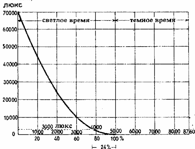
6. График годового распределения освещенности по числу часов и интенсивности (важно для назначения величины E_{нар} )
