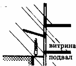
4. Устройство козырька над витриной, освещение которой обеспечивается призматическими стеклами. Освещение подвала через приямок с призматическими стеклами на уровне тротуара 1 - витрина; 2 - подвал
