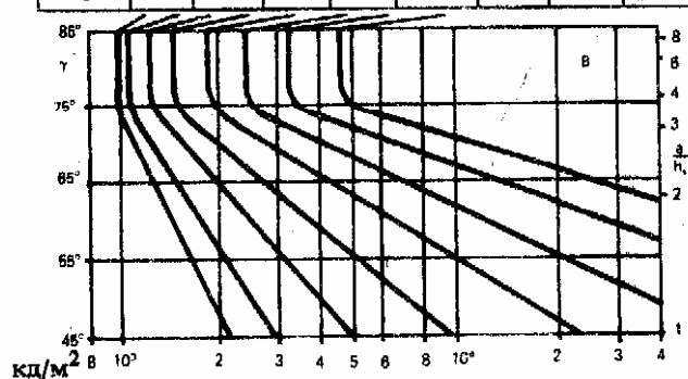
3. Кривые предельной яркости вытянутых квадратных и круглых светильников, с боковым светом, расположенных перпендикулярно направлению взгляда, например светильники в ванных
