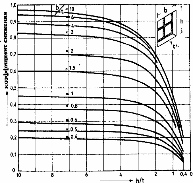
2. График для определения коэффициента снижения освещенности при глубоких оконных откосах
