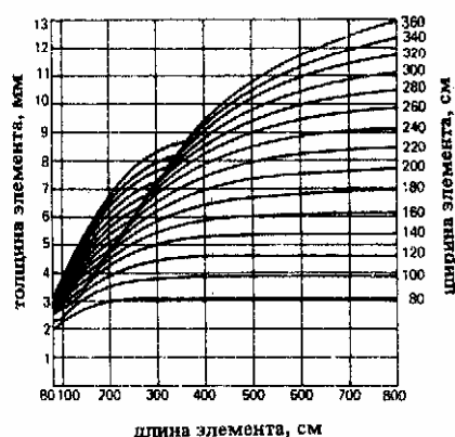
4. Диаграмма ветровых нагрузок для расчета толщины стекла изолирующих элементов по DIN 1055
