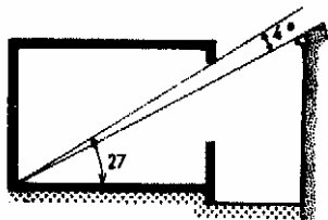
2. Угол падения луча света, образованный касательной наружной грани перемычки из самой дальней точки пола должен быть \geq 27^\circ ; угол свободного обзора из этой же точки \geq 4^\circ
