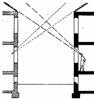
3. Из окон нижнего этажа должно быть видно небо
