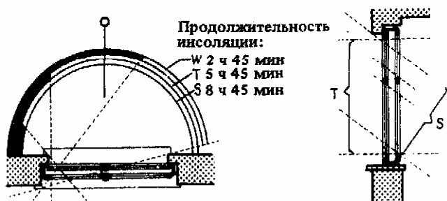
2. В окна, ориентированные на восток и на запад, во время равноденствия проникают горизонтальные лучи: к летнему солнцестоянию угол падения лучей увеличивается (рис. 3). Справа разрез
