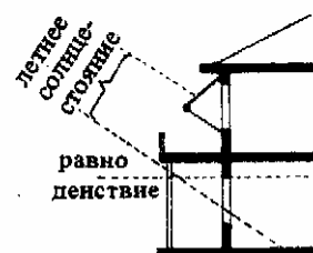
11. Восточный фасад. Полуденные солнечные лучи позволяют устраивать широкие, чаще всего защищенные от ветра террасы, не препятствующие инсоляции
