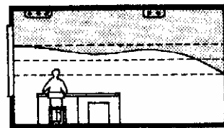
7. Кривая освещенности при наличии второго ряда ламп
