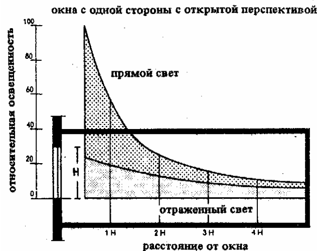
5. Удельный вес прямого и отраженного света и освещенности помещений
