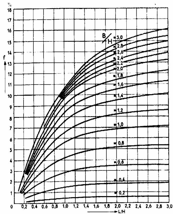
1. График для определения освещенности наружной поверхности окон во дворах (без учета затенения оконными откосами и отражения от стен противостоящих зданий)
