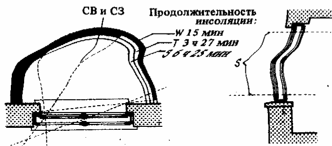
5. В окна северо-восточного и северо-западного фасадов солнечные лучи зимой не попадают, зато обеспечивается интенсивная инсоляция весной и осенью. Летом через них проникают горизонтальные лучи солнца. Справа разрез
