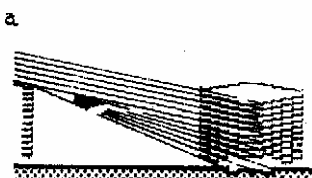
5. В больших зданиях ступенчатое расположение перекрытий с понижением отметок к середине может обеспечить естественное освещение на всю глубину помещений через высоко расположенные окна; в зависимости от назначения здания глубина корпуса может быть доведена до 30-60 м (запатентовано автором)
