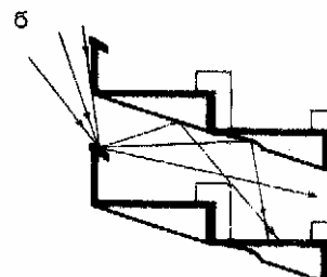
6. Разницу отметок перекрытия при больших пролетах между колоннами может быть использована для размещения прогонов. Неизбежные при этом наклонные потолки хорошо отражают свет; подоконник, интенсивно отражающий свет, способствует освещению потолка при падении света под большим углом
