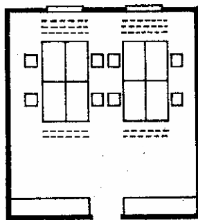
6. В глубоких помещениях второй ряд ламп размещают на \frac{2}{3} глубины помещения (рис. 7)
