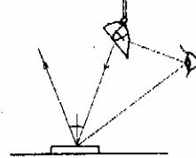
4. Угол падения световых лучей на зеркальную рабочую поверхность должен быть таким, чтобы не возникало слепящих лучей от обрабатываемых деталей
