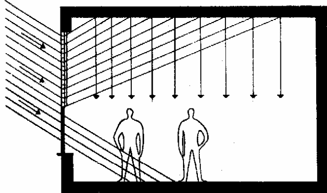
применение светопреломляющих стеклоблоков для более равномерного освещения
