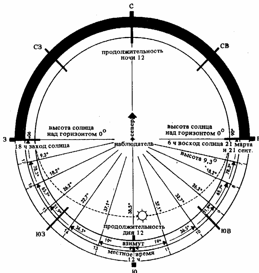
2. Траектория движения солнца в период зимнего солнцестояния (около 21 декабря) и осеннего равноденствия (около 21 сентября)
