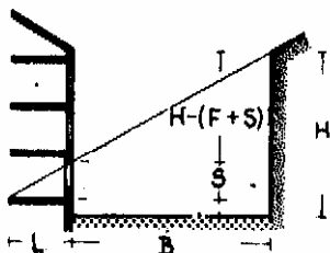
3. Определение естественного освещения по эмпирической формуле Кюстера; площадь L \geq 1/3-1/2 площади пола
