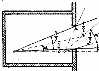
3. Свет падает под слишком малым углом. Наиболее освещенная точка расположена в глубине помещения
