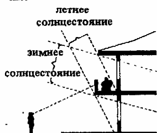
10. Южный фасад. Зимой теплые солнечные лучи проникают в глубину помещения. Летом окна и стены защищены от солнечного перегрева
