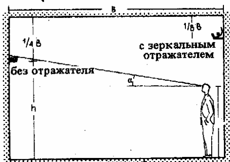
1. Скрытые за карнизом источники отраженного света
