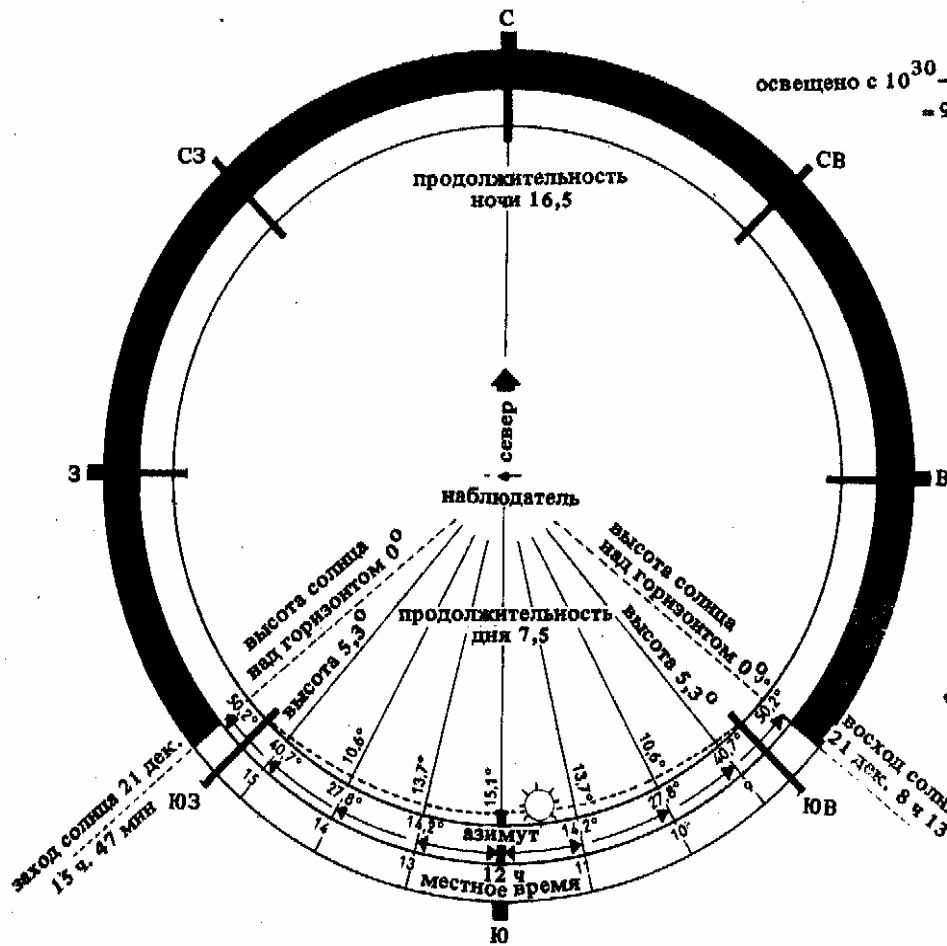
1. Траектория движения солнца в период зимнего солнцестояния (около 21 декабря) для самого короткого дня в году (31,5° северной широты, Дортмунд-Галле)
