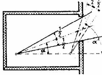
4. Свет падает под большим углом. Лучшая освещенность на рабочей плоскости (на высоте 1 м)
