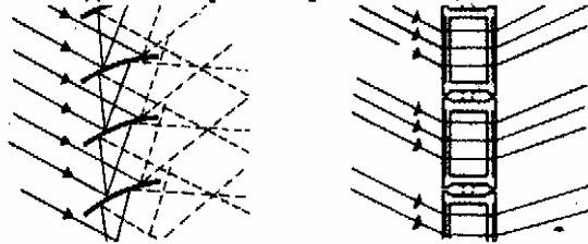
преломление света специальными стеклоблоками
