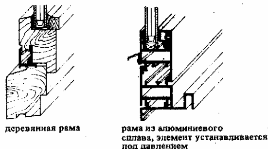
5. Установка стеклянных изолирующих элементов в оконную коробку
