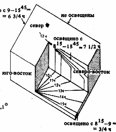
6. Зимнее солнцестояние. Северо-восточные фасады освещены в течение всего около часа, юго-восточные фасады оказываются в тени вскоре после 13 ч
