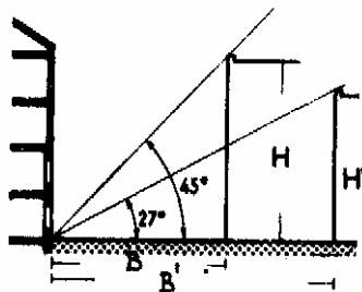
1. Нормальный профиль улицы. При угле 45^\circ B = H (в старом городском центре), при угле 27^\circ B = 2H (в районах новой застройки)
