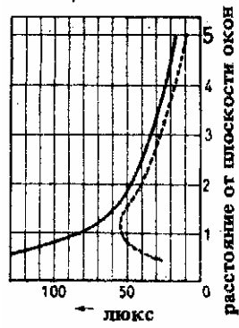
1. Кривые средней освещенности горизонтальной плоскости
