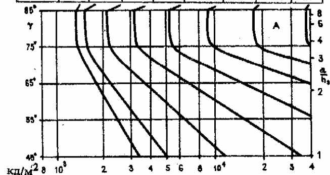
2. Кривые предельной яркости светильников с горизонтальной плоскостью светополучения; особенно пригодны для встроенных светильников. Все вытянутые светильники расположены параллельно направлению взгляда
