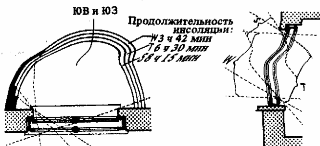
4. Окна юго-восточного и юго-западного фасадов обеспечивают летом и зимой инсоляцию помещения полуденными, глубоко проникающими лучами. Справа разрез
