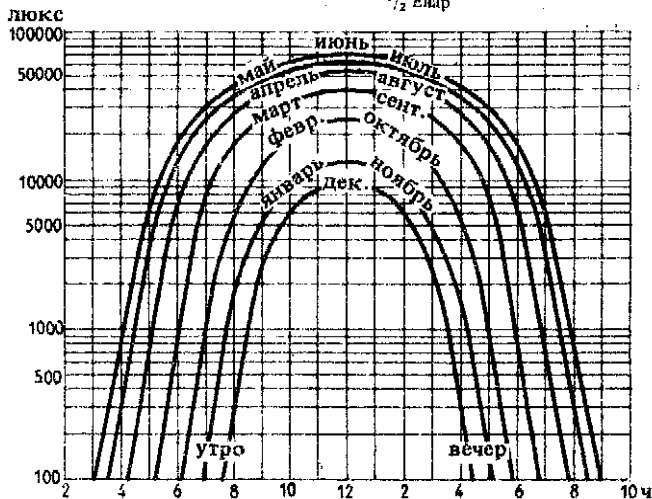
5. График суточного изменения средней освещенности горизонтальной поверхности на открытом воздухе (по среднемесячным данным метеорологической обсерватории в Потсдаме)
