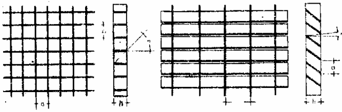
1. Прямоугольная решетка
