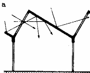
8. Шедовое или пилообразное покрытие создает более равномерную освещенность благодаря отражению света нижней поверхностью; при светлых крышах равномерность освещения повышается. Фонари не доводят до наружных стен здания
