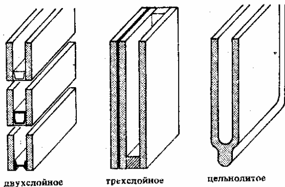
1. Конструкция изолирующего стекла
