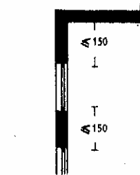
4. Расстояние от края остекления окон до боковой стены и между смежными окнами одного помещения не должно превышать 150 см
