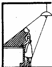
1. При установке светильника, освещающего рабочее место, следует учесть тень, отбрасываемую работником
