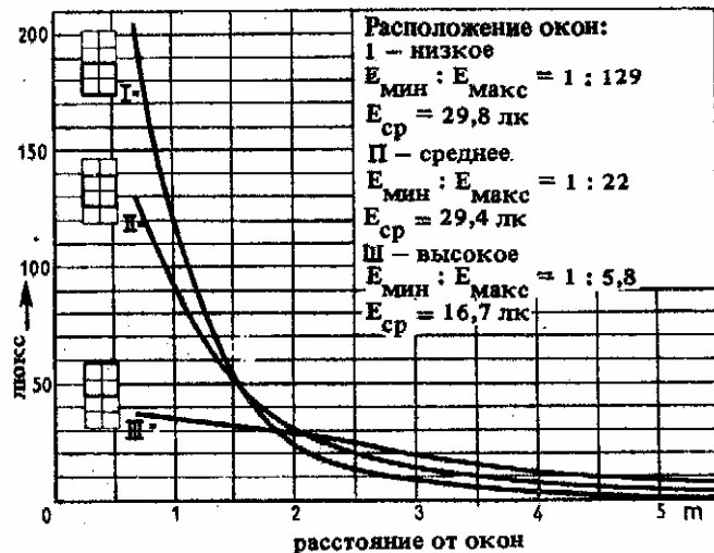
2. Чем выше размещены окна, тем светлее в глубине помещения и тем выше равномерность освещения
